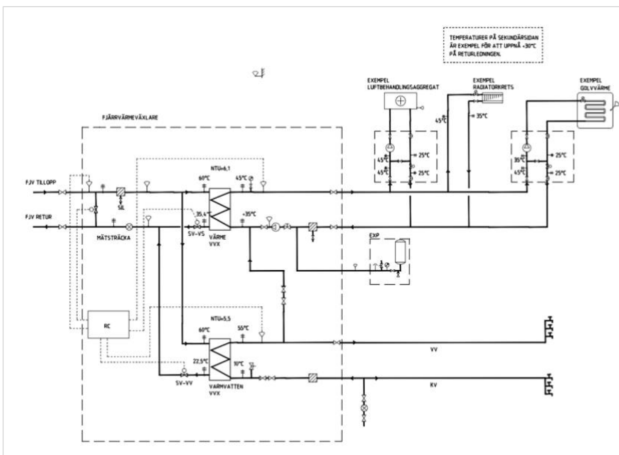
Figur 3. Kopplingsprincip för fjärrvärmväxlare villa/radhus ansluten till 2-rörssystem
