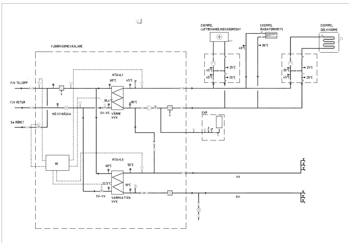
Figur 3. Kopplingsprincip för fjärrvärmeväxlare villa/radhus ansluten till 3-rörssystem
