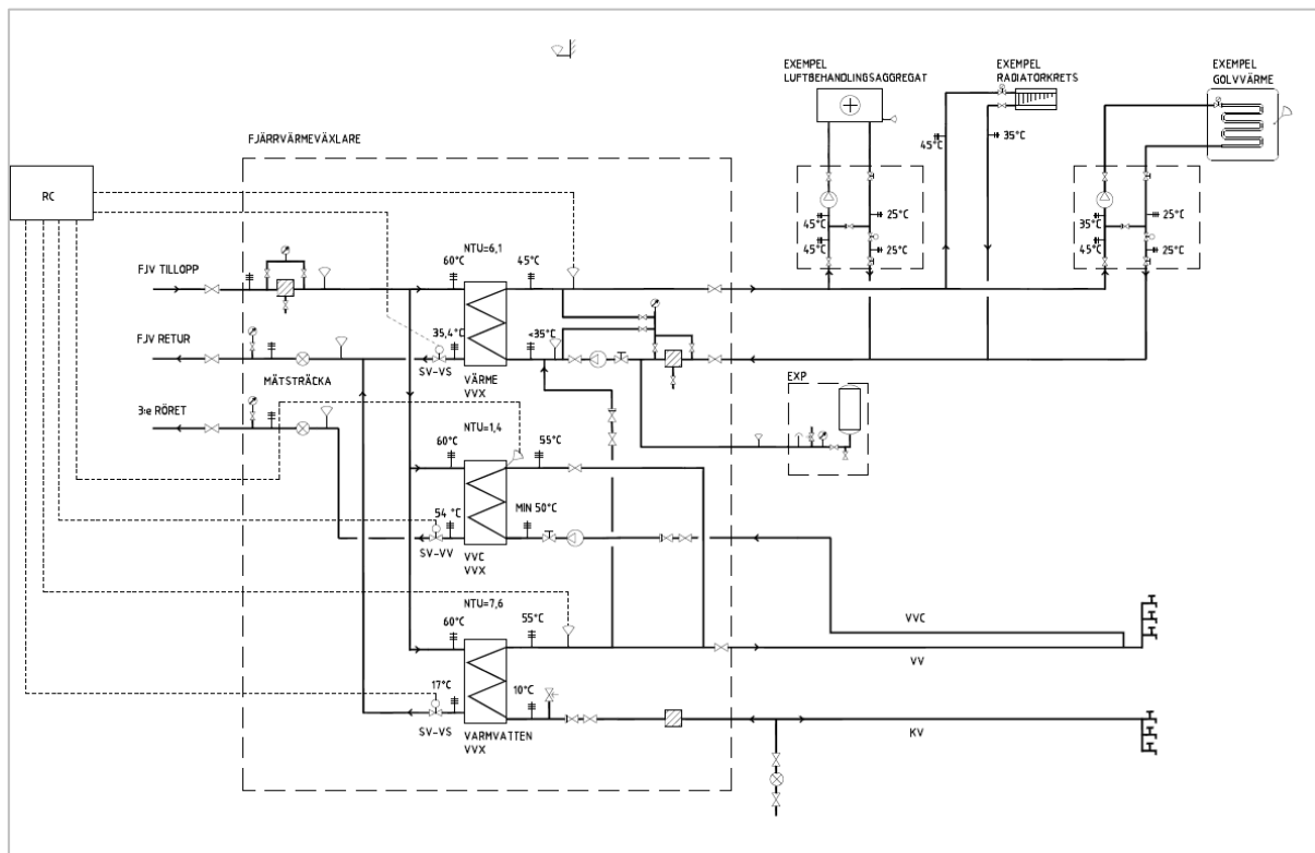
Figur 4. Kopplingsprincip för fjärrvärmväxlare flerbostadshus ansluten till 3-rörssystem.
