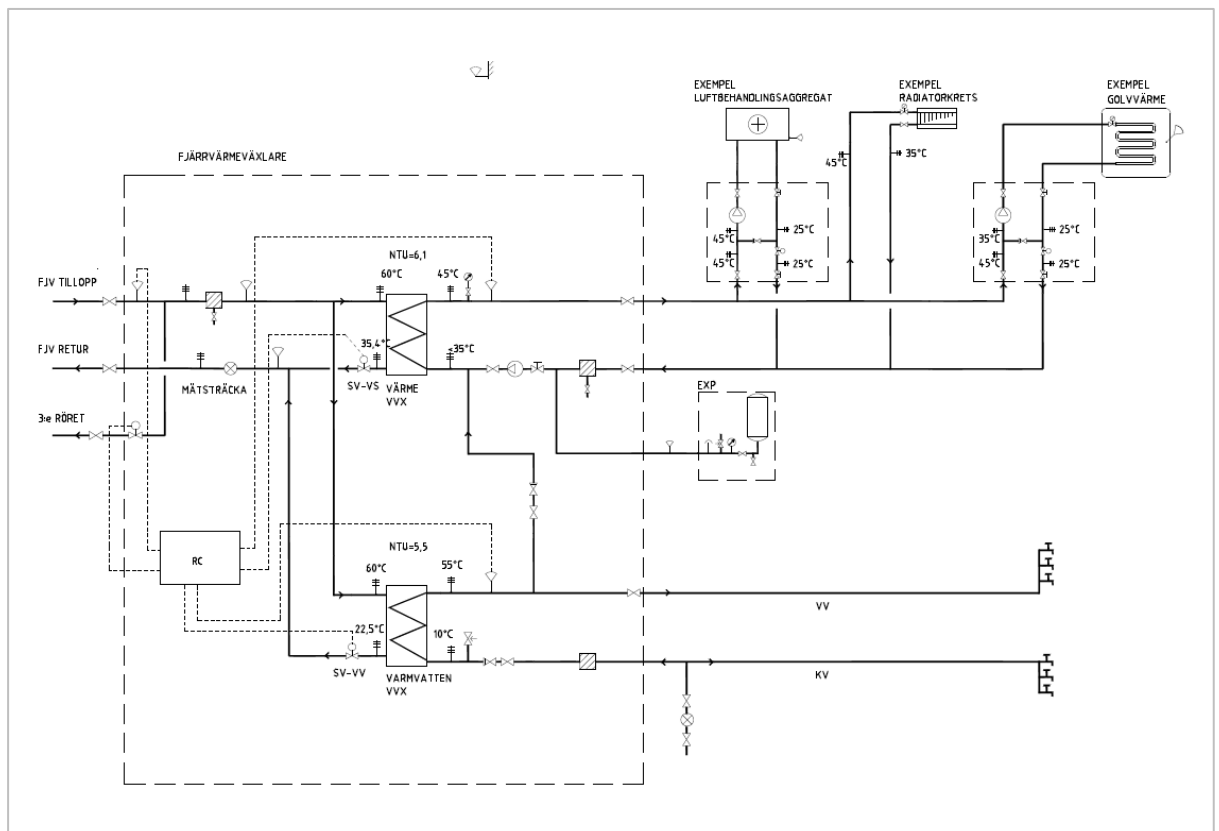
Figur 3. Kopplingsprincip för fjärrvärmeväxlare villa/radhus ansluten till 3-rörssystem
